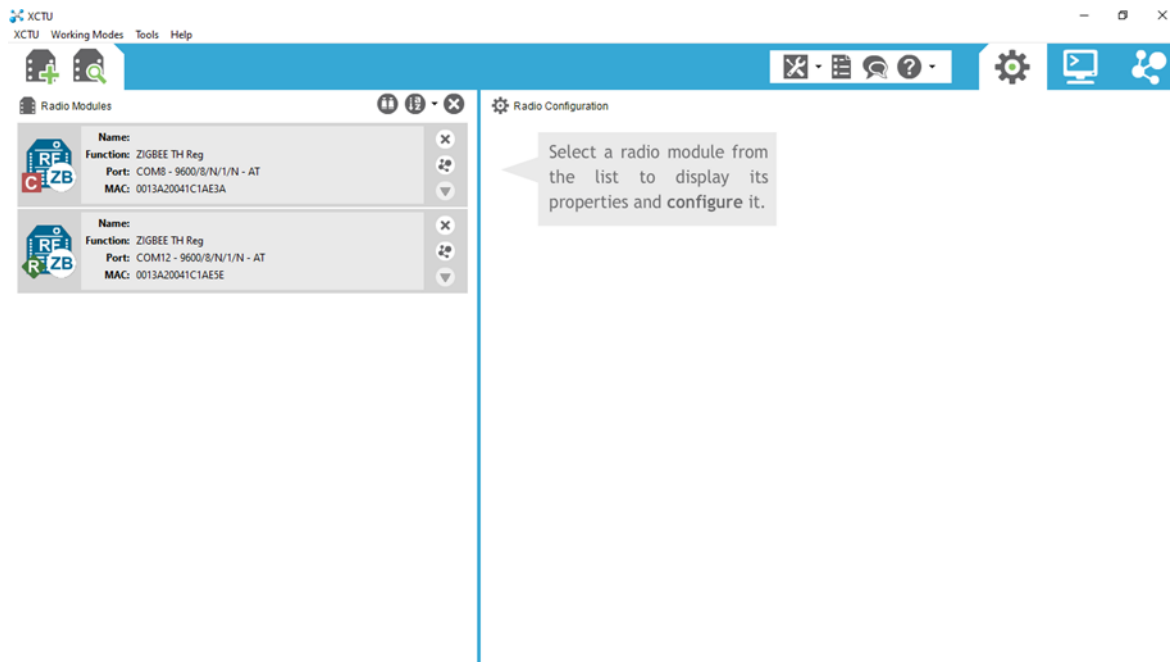
Fig. 6 Módulos XBee reconocidos en XCTU.
